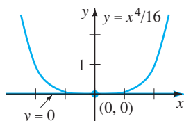
FIGURA 1.2.5 Dos soluciones del mismo PVI.
