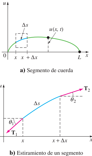
FIGURA 12.2.2 Cuerda flexible anclada en x = 0 y en x = L .
