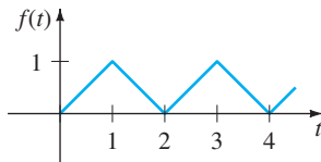
función triangular
