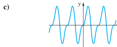
FIGURA 4.4.3 Curva solución.
