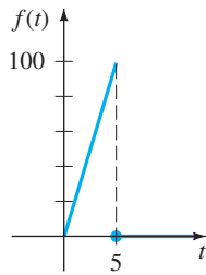
FIGURA 7.3.5 La función es f(t) = 20t - 20t\mathcal{U}(t-5) .
