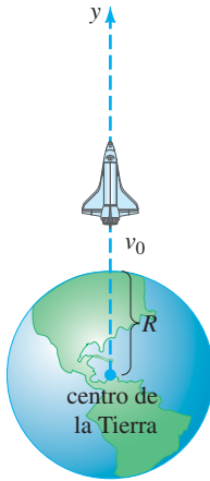
FIGURA 5.3.5 La distancia al cohete es grande comparada con R .
