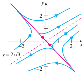
FIGURA 10.2.6 Punto silla.
